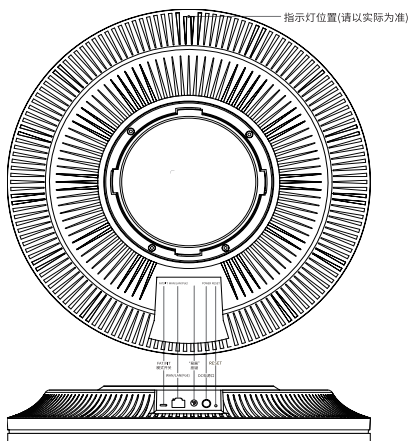
图1-2 底面和侧面示意图
