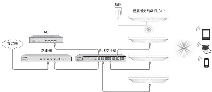
图4-8 典型应用拓扑图-易展分布式无线组网
