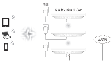
图4-3 典型应用拓扑图-易展分布式无线组网（二）
