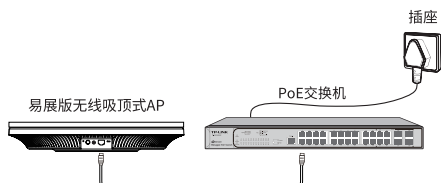
图2-1 PoE供电示意图示
