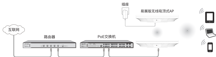
图4-2 典型应用拓扑图-易展分布式无线组网(一)
